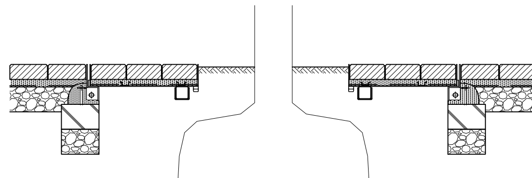
施工参考図
